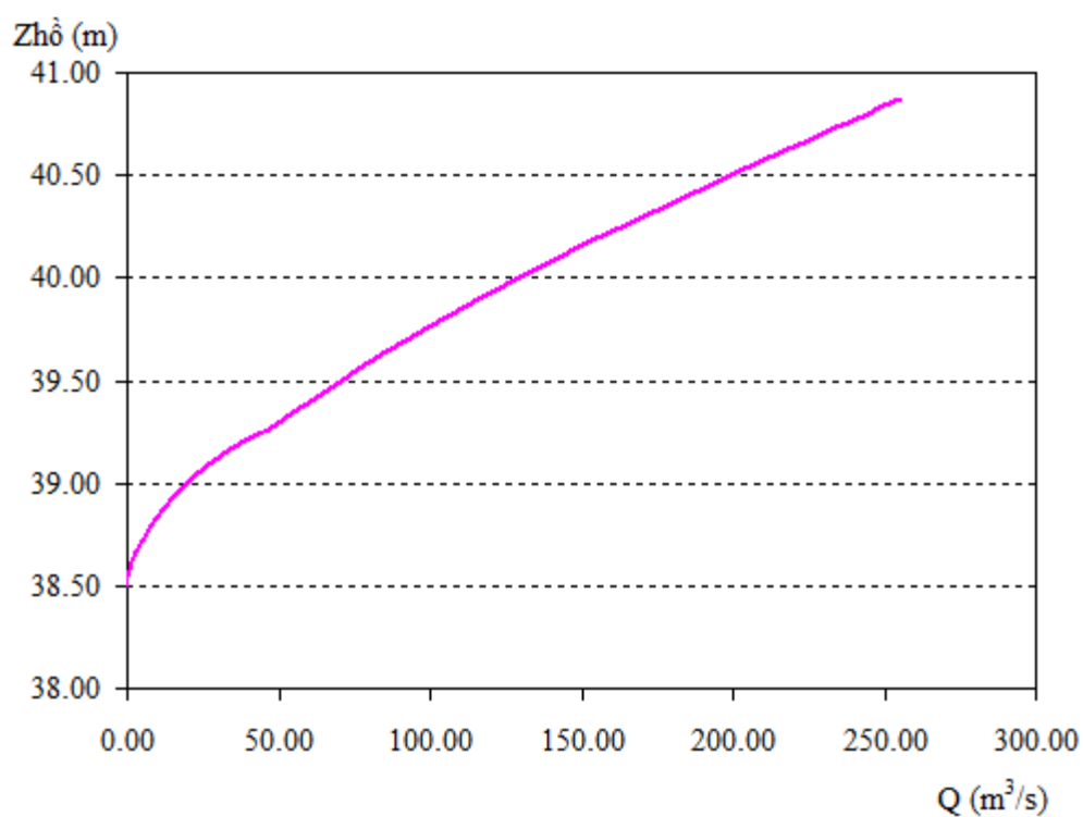
QUAN HỆ MỰC NƯỚC - LƯU LƯỢNG XẢ QUA TRÀN XẢ LŨ (Ngưỡng 38,50m)
