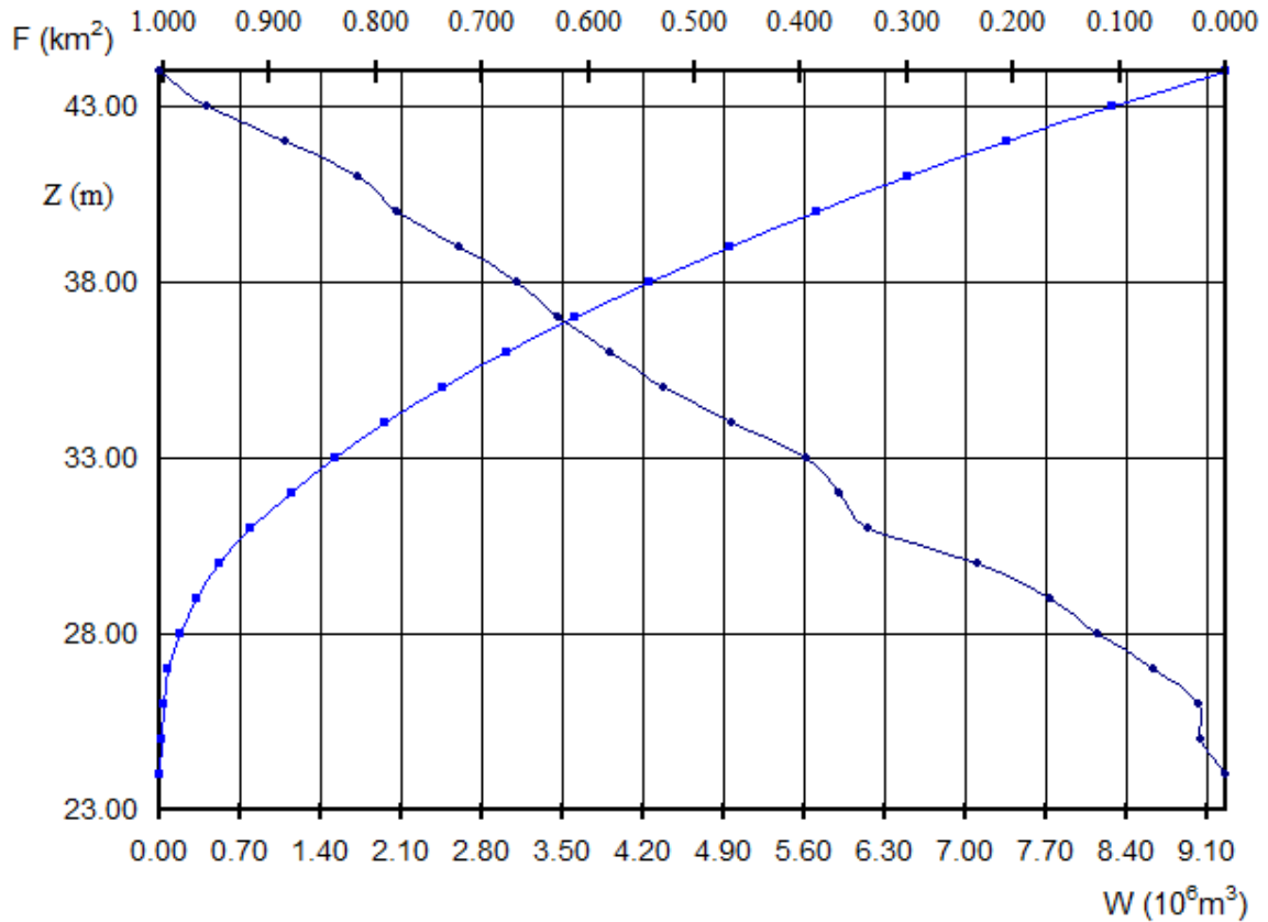
5. Bảng quan hệ lòng hồ Z \sim F \sim W
