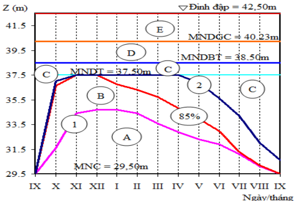
BIỂU ĐỒ ĐIỀU PHỐI HỒ CHỨA NƯỚC KHE CÒ
