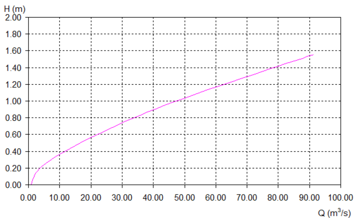
QUAN HỆ CỘT NƯỚC TRÀN - LƯU LƯỢNG XẢ QUA TRÀN XẢ LŨ (Ngưỡng tràn = 39,50m)
