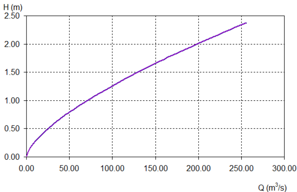
QUAN HỆ CỘT NƯỚC TRÀN - LƯU LƯỢNG XẢ QUA TRÀN XẢ LŨ (Ngưỡng tràn = 39,50m)
