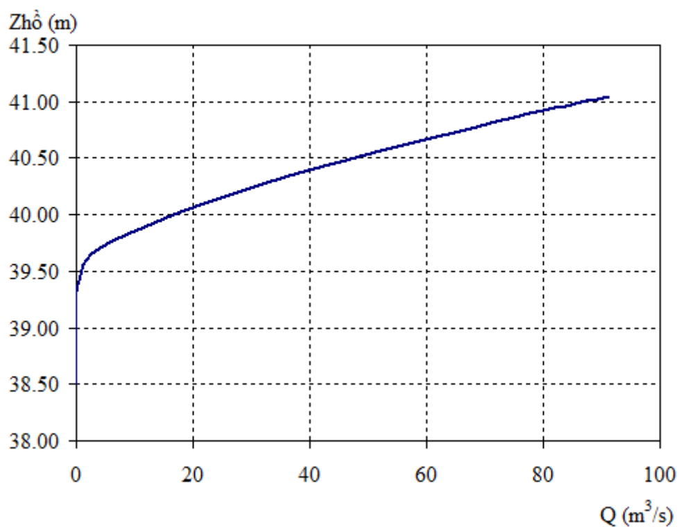
QUAN HỆ MỰC NƯỚC - LƯU LƯỢNG XẢ QUA TRÀN XẢ LŨ (Ngưỡng 39,50m)
